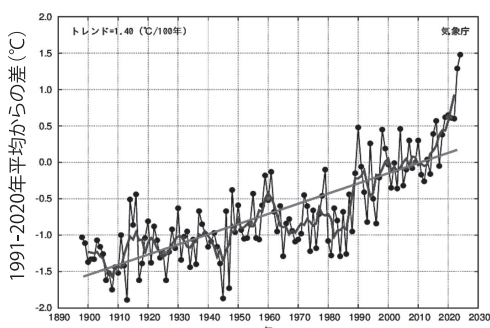
1890年～2024年 日本の年平均気温偏差(気象庁)
